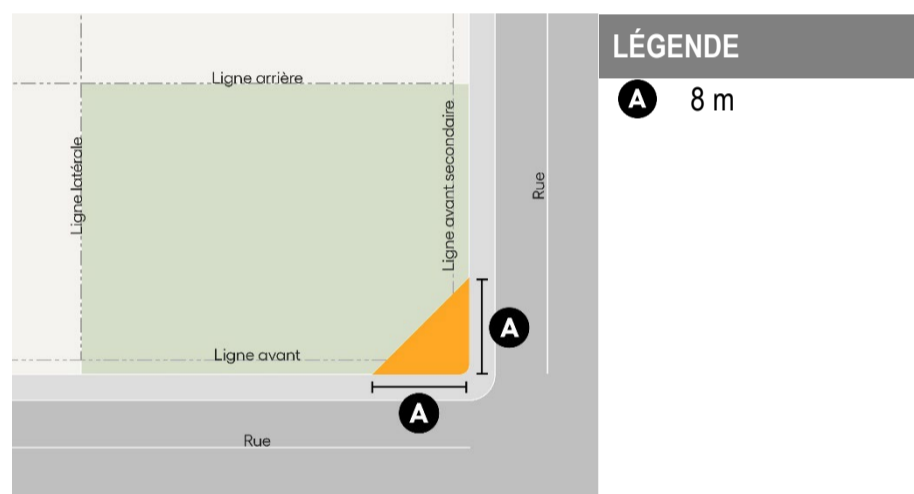
FIGURE 3 - Triangle de visibilité
